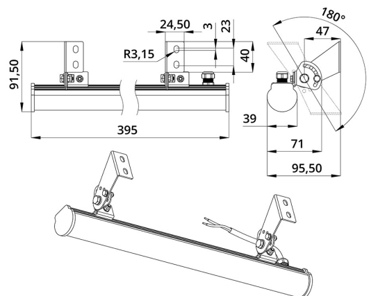
Габаритный чертеж
