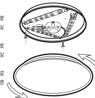
Рис 2. Подключение светильника PPB BREEZE
