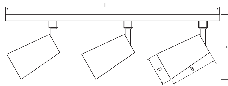
Рис.1 Комплект PTR 1508
