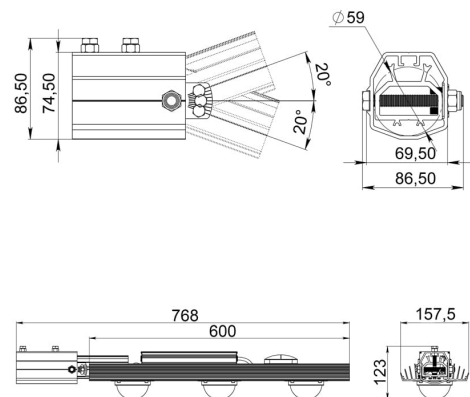
Габаритный чертеж
