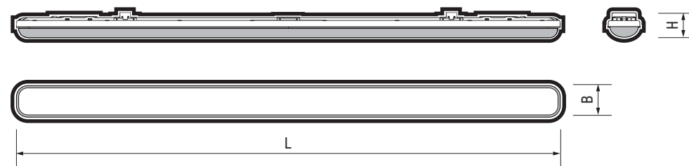
Рис.1 Светильник PWP-C5 PRO
