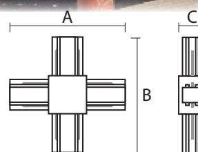
Коннектор X-образный
